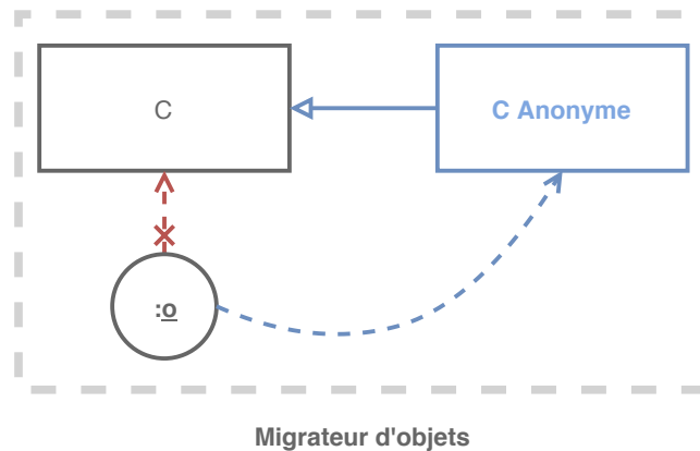
FIGURE 4.8 – À partir d'un couple \{objet, classe\ anonyme\} , le migrateur brise le lien entre l'objet et sa classe d'origine, et lie l'objet à la classe anonyme qui devient sa classe courante. Les états de l'objet sont migrés vers sa nouvelle structure, et les nouveaux états éventuels de l'objet sont initialisés.
